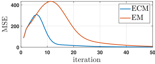
FIGURE 2 : MSE de la position et de l'orientation \Phi au cours des itérations.
