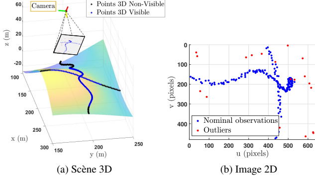
FIGURE 1 : Nuage de points 3D du scénario étudié, présenté dans la partie 4 (gauche), et nuage de points 2D distinguant les valeurs aberrantes en rouge et non aberrantes en bleu (droite).
