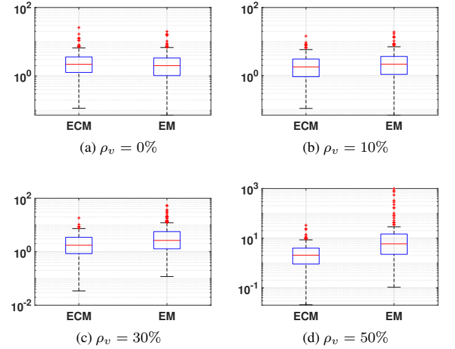
FIGURE 3 : Boxplots des MSE du vecteur (position, orientation) \Phi pour différentes valeurs de la proportion de données aberrantes \rho_v .
