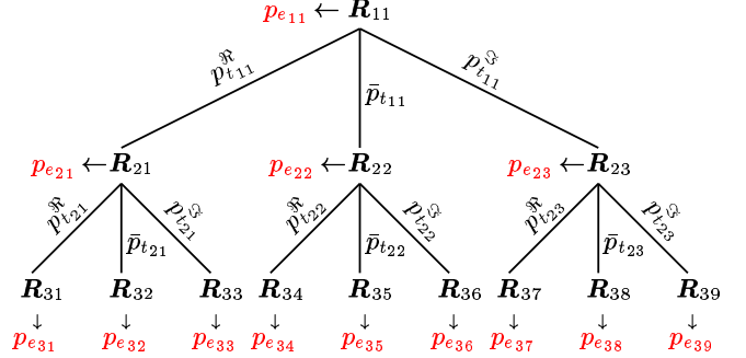
FIG. 2: Représentation en « arbre » des matrices de covariance \mathbf{R}_{ij} (sur les « nœuds ») et des probabilités de transition p_t (sur les « branches ») pour 3 niveaux (3 émetteurs classés dans l'ordre utilisé par le récepteur V-BLAST). À chaque \mathbf{R}_{ij} correspond le TEB p_{e_{ij}} .
