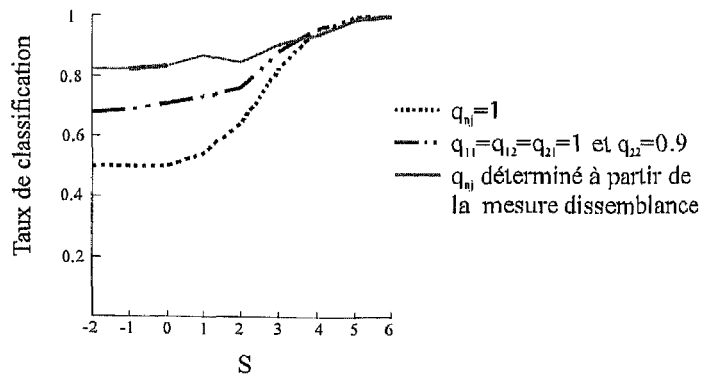
Figure 4. – Evolution du taux de classification en fonction du signal S
