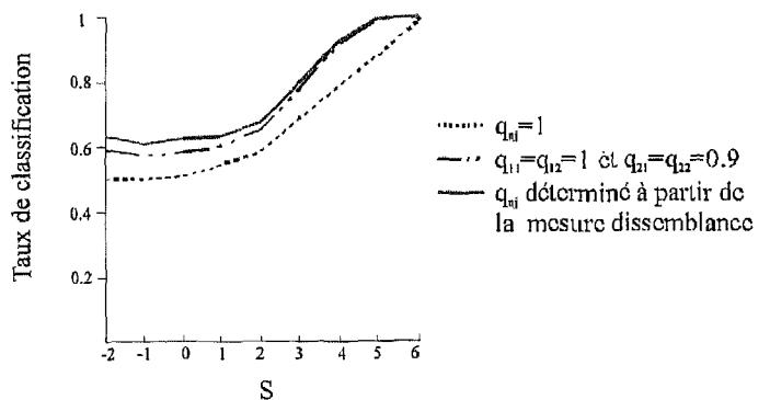
Figure 6. – Evolution du taux de classification en fonction du signal S
