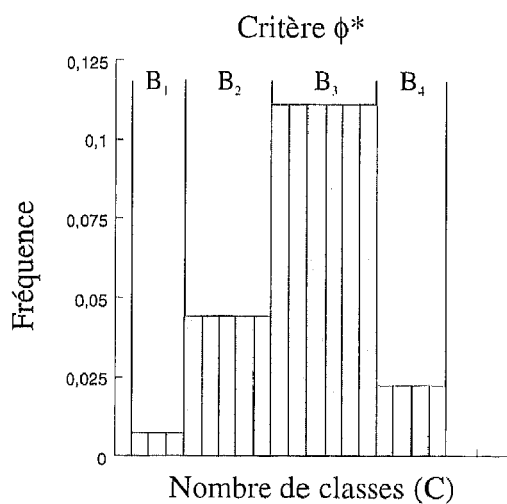
Figure 3. – Histogrammes optimaux selon le critère d'information.
