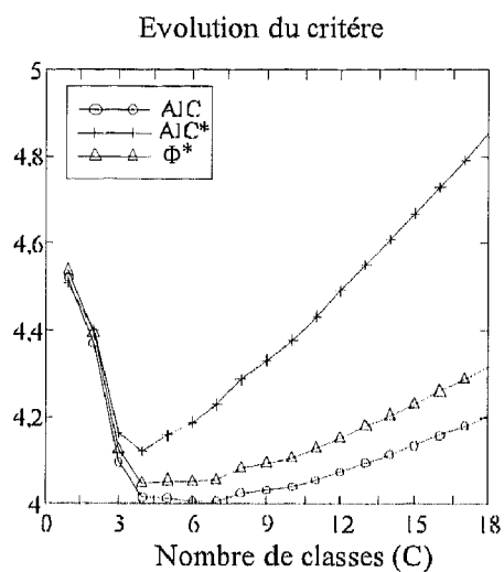
Figure 2. – Evolution des critères d'information en fonction du nombre de classe.
