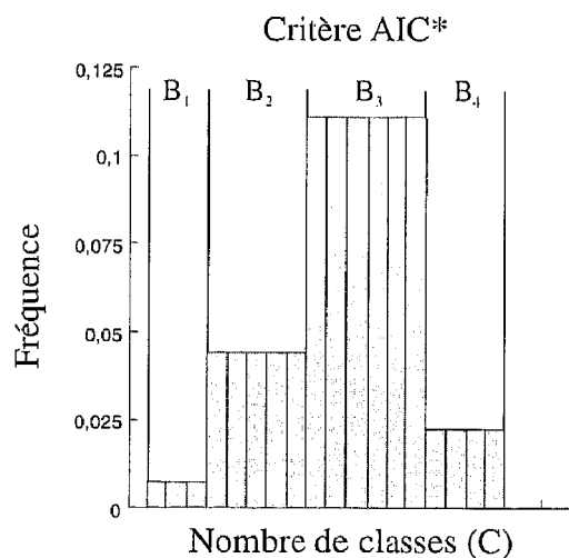
Figure 2. – Evolution des critères d'information en fonction du nombre de classe.
