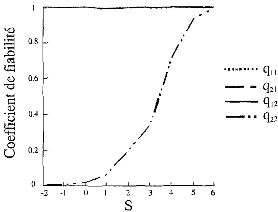
Figure 5. – Evolution des coefficients de fiabilité déterminés à l'aide de la distance de Hellinger en fonction du signal S
