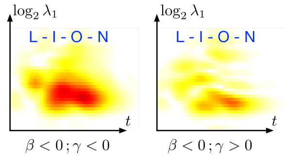
FIGURE 3 – En haut, un scalogramme x_1(t, \log_2 \lambda_1) du mot anglais lion (prononcé /laɪən/). En bas, coefficients de scattering de x_2(t, \log_2 \lambda_1, \log_2 \lambda_2) en fonction du temps t et de la log-fréquence \log_2 \lambda_1 , pour \lambda_2 = (\alpha, \beta, \gamma) fixé avec \alpha^{-1} = 120 ms, \beta^{-1} = \pm 1 octave, \gamma^{-1} = \pm 4 octaves. La clarté est inversement proportionnelle à l'amplitude des coefficients.
