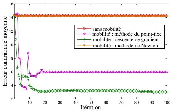
FIGURE 2 – Performances des méthodes proposées.
