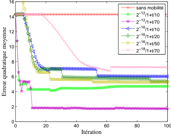
FIGURE 1 – Evolution de l’erreur quadratique moyenne de la méthode de descente de gradient pour différentes valeurs du pas \eta_t .
