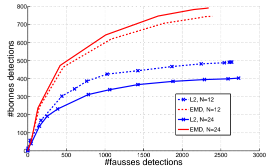
FIG. 2 – Comparaison des distances L^2 et EMD.
