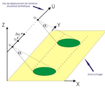
Figure 1: Système d'acquisition de données RSO
