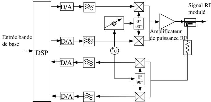
FIG. 1 – Schéma de principe d'un système de pré-distorsion en bande de base
