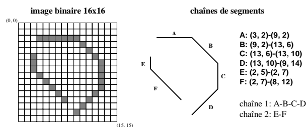
Figure 1: Exemple de chaînage de contours
