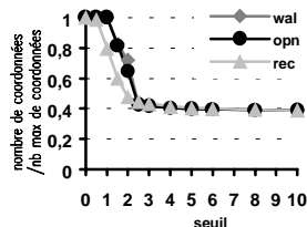
Figure 11: Evolution du nombre de coordonnées
