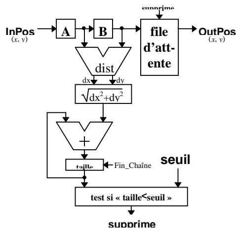
Figure 17: Architecture de l'élimination des petites chaînes
