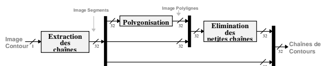
Figure 2: Synoptique du chaînage de contours
