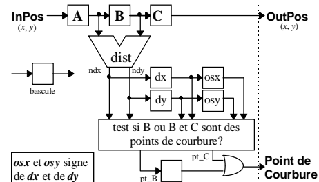
Figure 14: Architecture de la recherche des points de courbure
