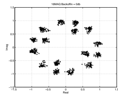
FIG. 3 — Dispersion de la constellation reçue.
