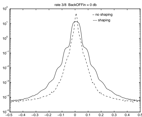
FIG. 5 — Réduction de l'élargissement spectral.
