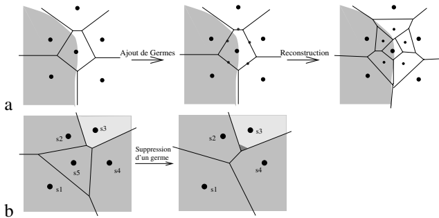
FIG. 1 — Illustration du processus de division (a) et de fusion (b).
