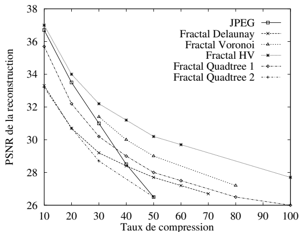
FIG. 7 — Comportement de différents algorithmes de compression sur l'image lena 512 \times 512 .
