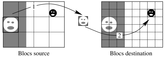
FIG. 2 — L'identification d'un collage, se fait par la connaissance d'un bloc destination et du bloc source qui l'approxime le mieux au travers d'une fonction affine. Cette fonction est autant que possible contractante sur \mathbb{R}^2 (1), mais agit également sur l'espace des luminances (2).
