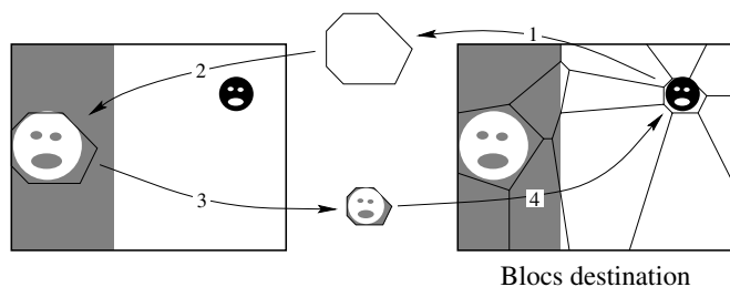
FIG. 3 — La structure du polygone destination est extraite et dilatée d'un facteur d (1) puis positionnée sur la zone permettant le meilleur collage (2). Le polygone source ainsi formé est contracté d'un facteur d (3) et sa luminance est modifiée par une fonction affine (4).
